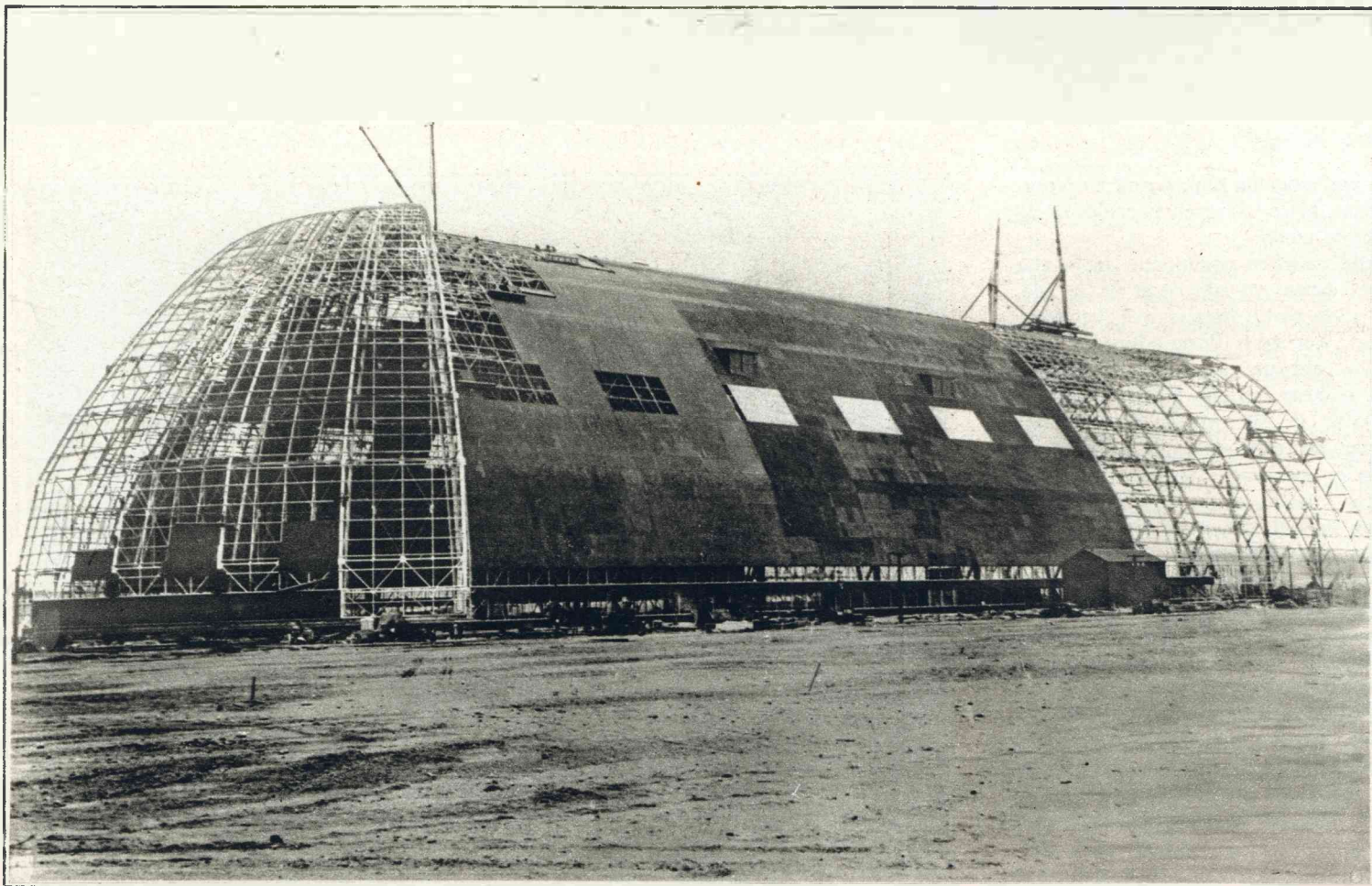
AMERIKAANSCH ZEPPELINS. In Akron (Ohio) is men begonnen aan den bouw van de reusachtige hall voor de nieuwe luchtschepen, die men in Amerika gaat bouwen. Deze luchtschepen zullen, naar verluidt, bijna tweemaal zoo groot zijn als de Duitsche Graf Zeppelin.
