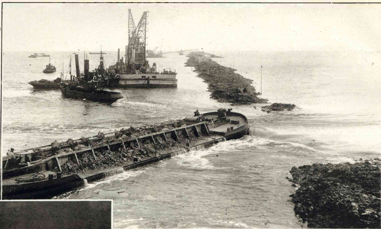
HET SLUITGAT in den dam tusschen Wieringen en Medemblik wordt gedicht. De foto is genomen uit een der grijpkranen. Een zgn. onderlosser laat zijn inhoud op den bodem der zee zinken.
