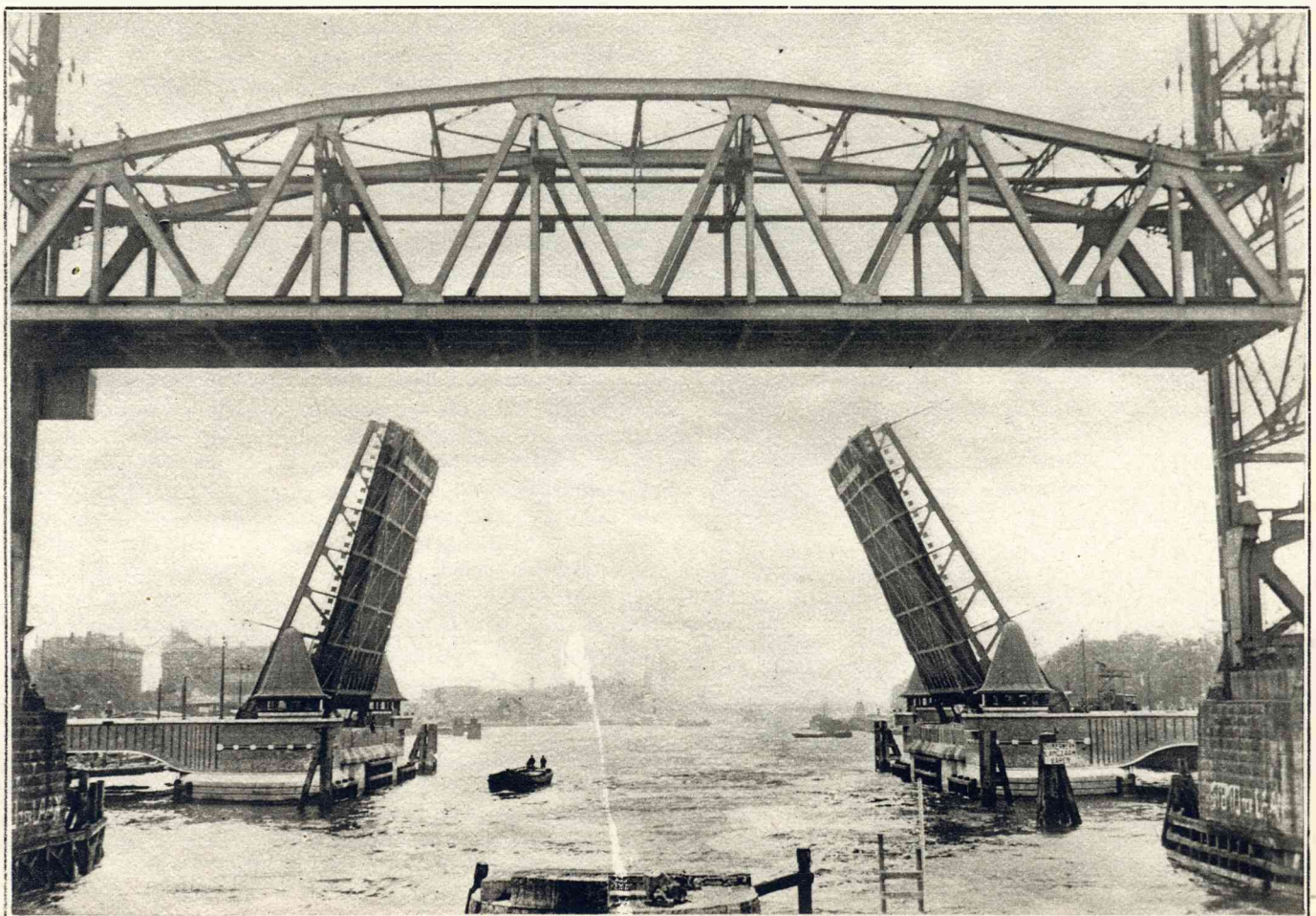
DE NIEUWE KONINGINNEBRUG te Rotterdam, die door Z.Exc. Minister mr. J. B. Kan officieel is opengesteld voor het verkeer, in geopen-den toestand.
