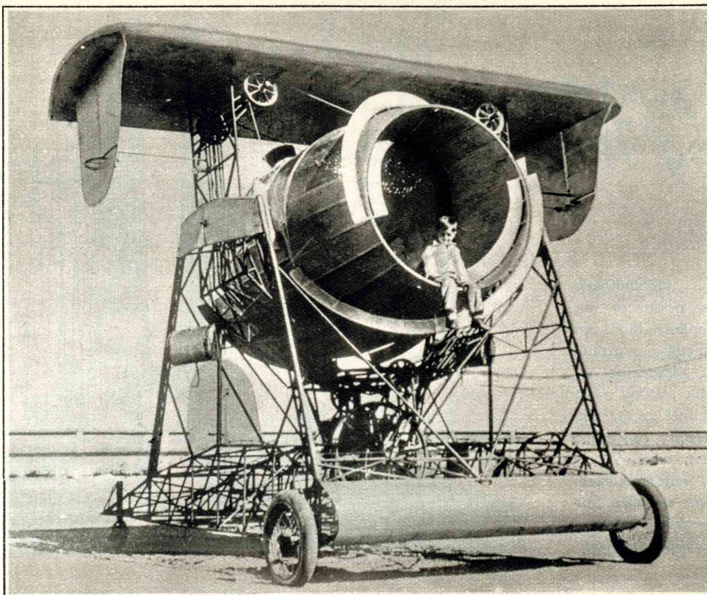
WEER 'N NIEUW model vliegtuig is geconstrueerd door Paul Maiworm in Californië. Hij vertrouwt een snelheid van 60 mijl per uur te bereiken door een snel draaiende hollen cylinder, die de schroef vervangt.
