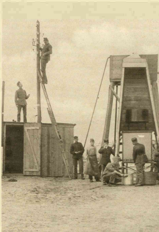
MODERNE GEMAKKEN. Het kamp beschikt over een „electrische centrale” en een motorisch gedreven waterleiding, dus over meer dan menig dorp beschikken kan.
