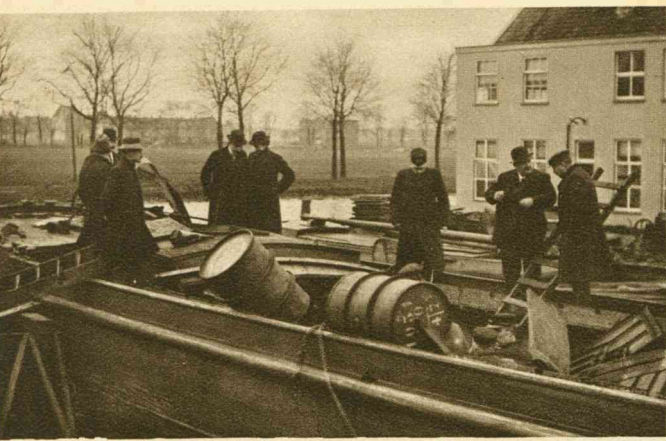
Een dezer dagen is een ijzeren pakschuit, die op de helling bij de firma v. d. Straaten en v. d. Brink aan den Trekvlut tusschen Den Haag en Rijswijk lag, bij het aanzetten van den motor uit elkaar gesprongen. Een werkman werd gedood, vier andere ernstig gewond.
